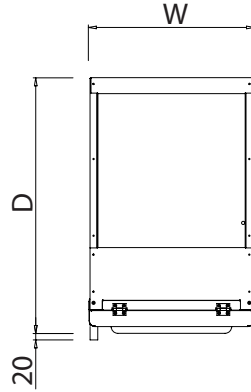
평면 / TOP VIEW
