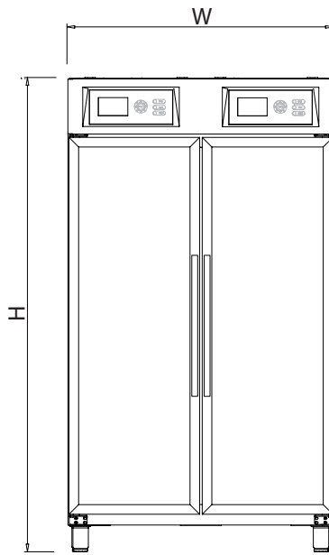
정면 / FRONT VIEW
