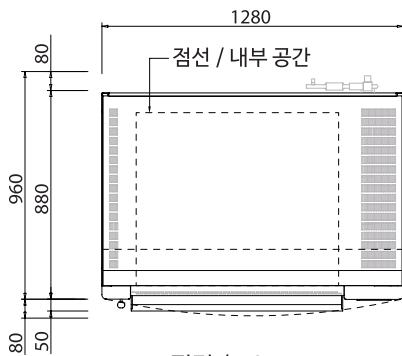
평면 / TOP VIEW
