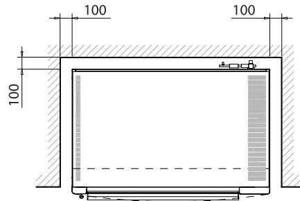
평면 / 설치 시 벽체와의 간격
