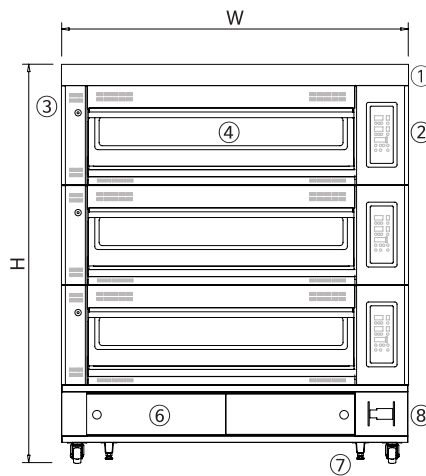
정면 / FRONT VIEW
