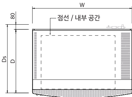
평면 / TOP VIEW
