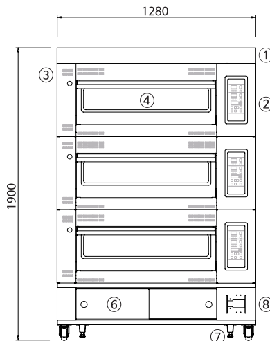
정면 / FRONT VIEW
